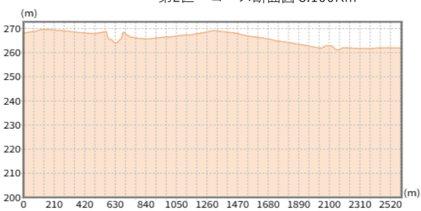
第4区 コース断面図 2.600Km
