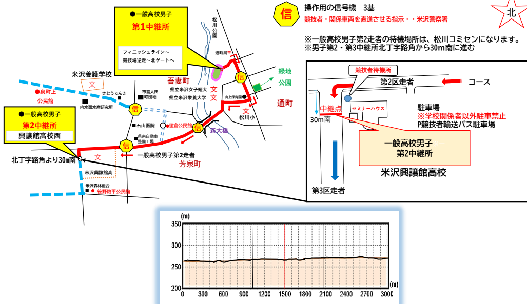
第2区 縦断面図
