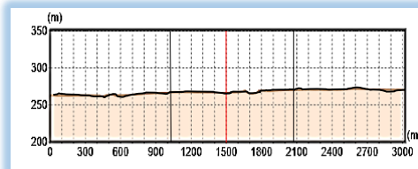
第2区 縦断面図
