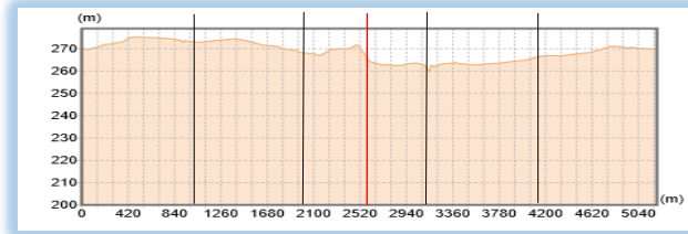
第3区 縦断面図
